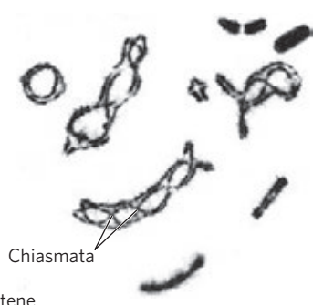
Diplotene
