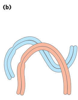
Leptotene
