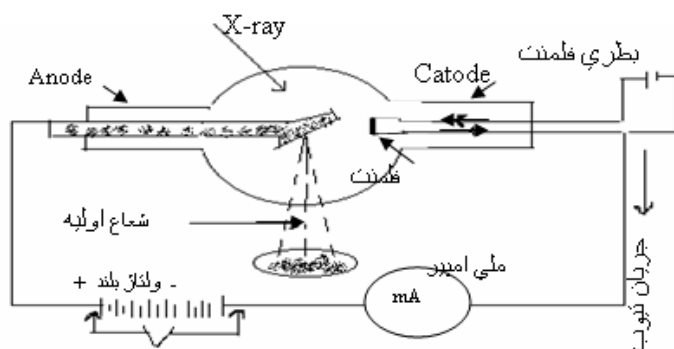
شکل (3-9) شمایی تیوب ساده کولیدج
