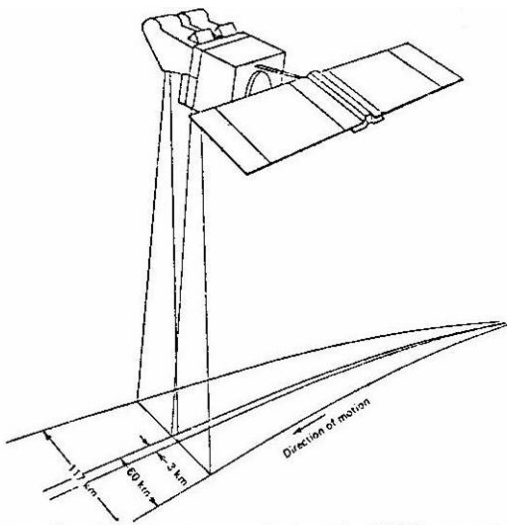
نگاره ۱۶-۱- اهداف اصلی از ارسال ماهواره اسپات عبارتست از : پونشن زمینی HRV اسپات موقعی که دو سنجنده پهلو به پهلو سطح زمین را بپوشانند. (انتباس از انتشارات سازمان فضایی فرانسه CNES) بکار می‌کنند. (انتباس از انتشارات سازمان فضایی فرانسه CNES)
