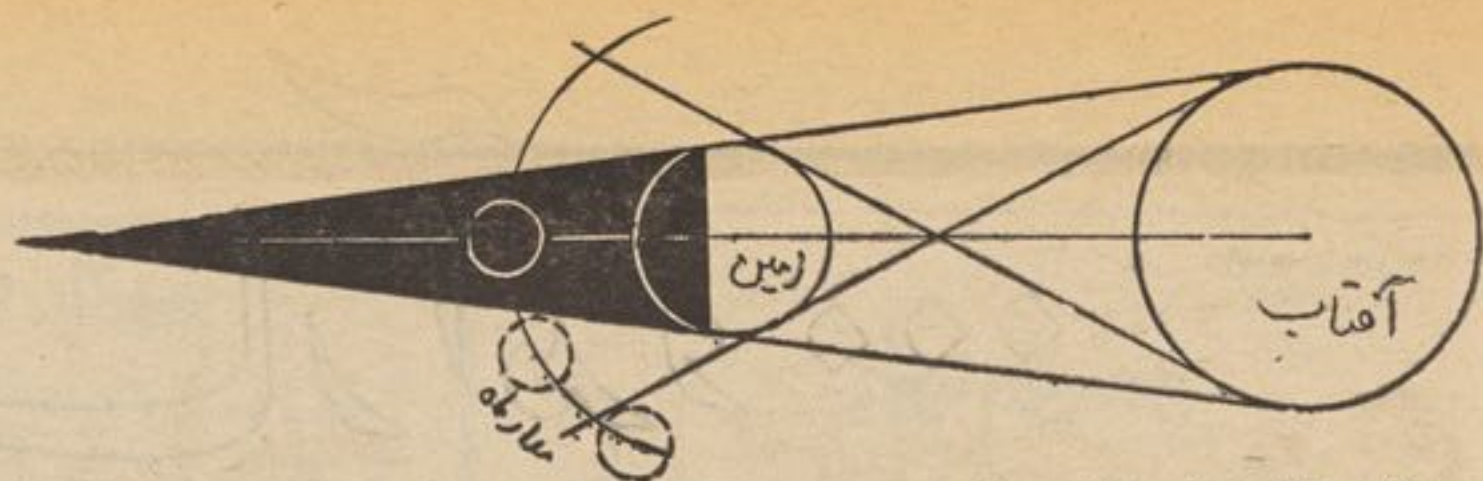
وقتی كه زمين در بين آفتاب و ماه حایل شود خسوف رخ مي دهد
