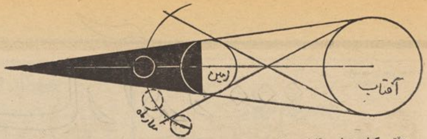
وقتي كه زمين در بين آفتاب و ماه حائل شود خسوف رخ ميدهد
