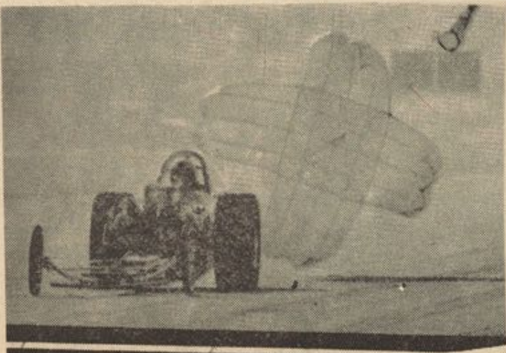
پارا شوت مخصوص كه در عقب موتر قرار دارد در توقف دادن موتر كمك ميكند .
