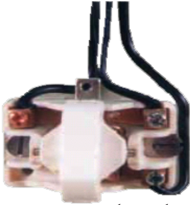
شکل (۲-۳) د راني ډوله تبدیل سویچ
