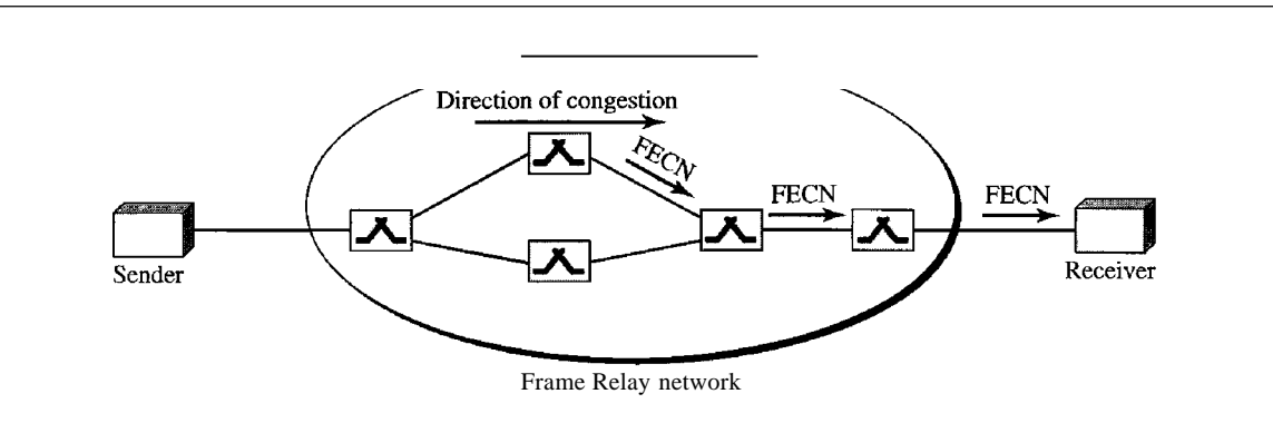
Figure 24.13 FECN
