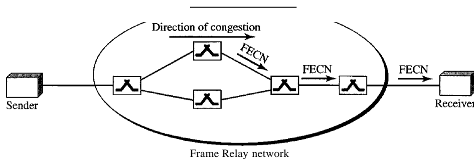
Figure 24.13 FECN
