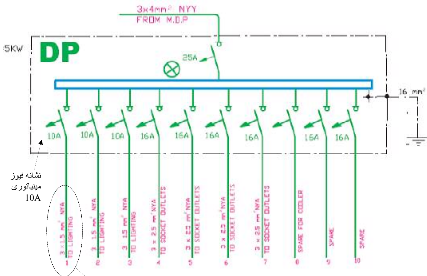
خط شماره یک تابلو سه سیم با مقطع 1.5 به سمت روشنایی (TO LIGHTING)
