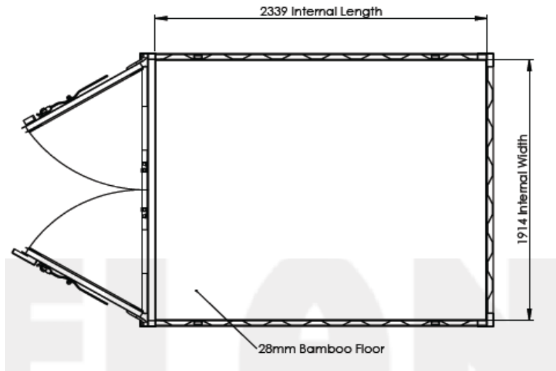
پلان کانتینر ۸ فت مینی
