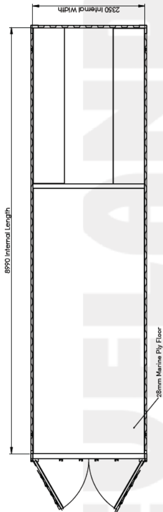
پلان کانتینر ۳۰ فوت
