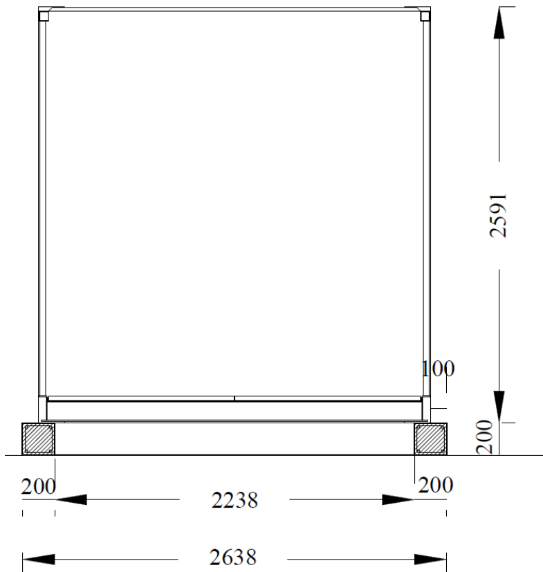
د کانتینر له پاره د کانکریت چوکاټ ۲۰۰ x ۲۰۰ ملی متر پرېک، نېټه ۱:۳
