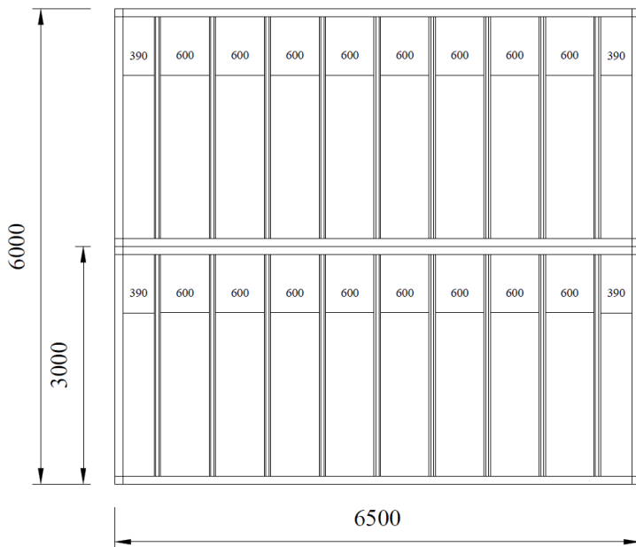
د تی آی ام کانکس غولی اسکلیت بندی پلان
