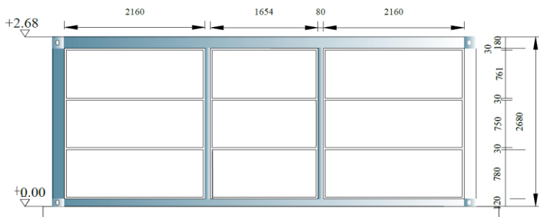
د تی آی ام کانکس دپوال اسکلیت بندی پلان
