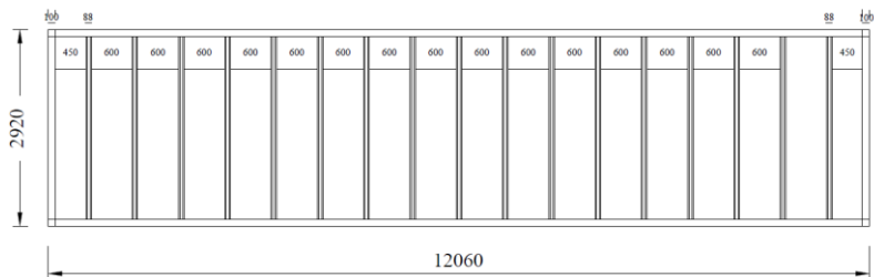
د تی آی ام حمامونو لرونکي کانتینر د غولي اسکلیټ بندۍ پلان
