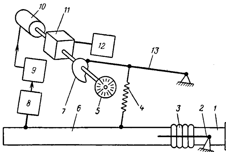
شیمای داتچیک (اندیکاتور) جبران کننده کثافت سنج وزنی
