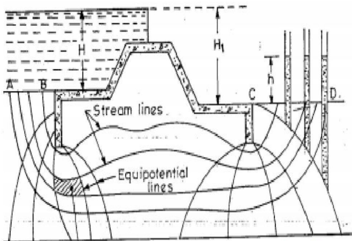
3.7 شکل: د خوسلا تيوري په بند کې رامنځته کېدونکې Piping ښايي.
