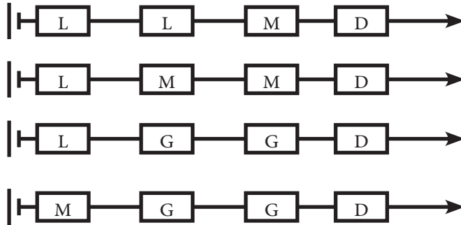
(۴-۶) شکل د استقرار ډول الف ( د تولید د عملیې پر اساس ب) د محصول د دستگاوو د ډول پر اساس L فرز (M) سنگ زني (G) ومته (D)
