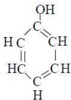
فینول
