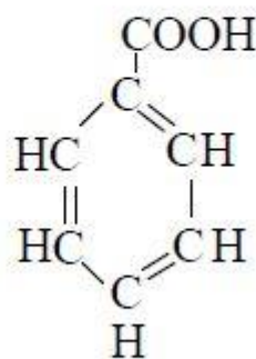
بنزوئيټک اسيد
