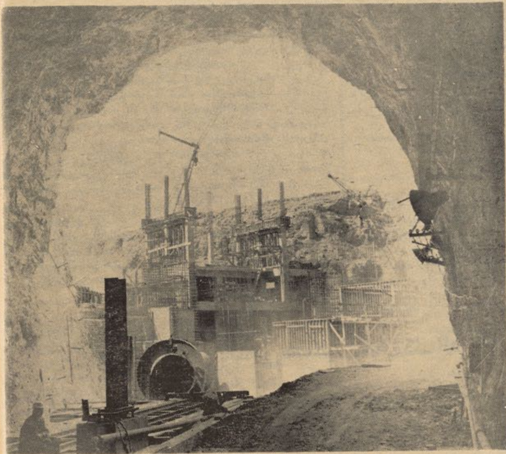
دور نمای دستگاه تو لیدی برق کجکی (پاور هوس) از داخل تونل
