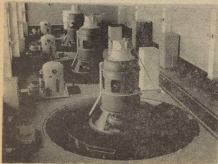
توربین چهارم دستگاه نغلو
