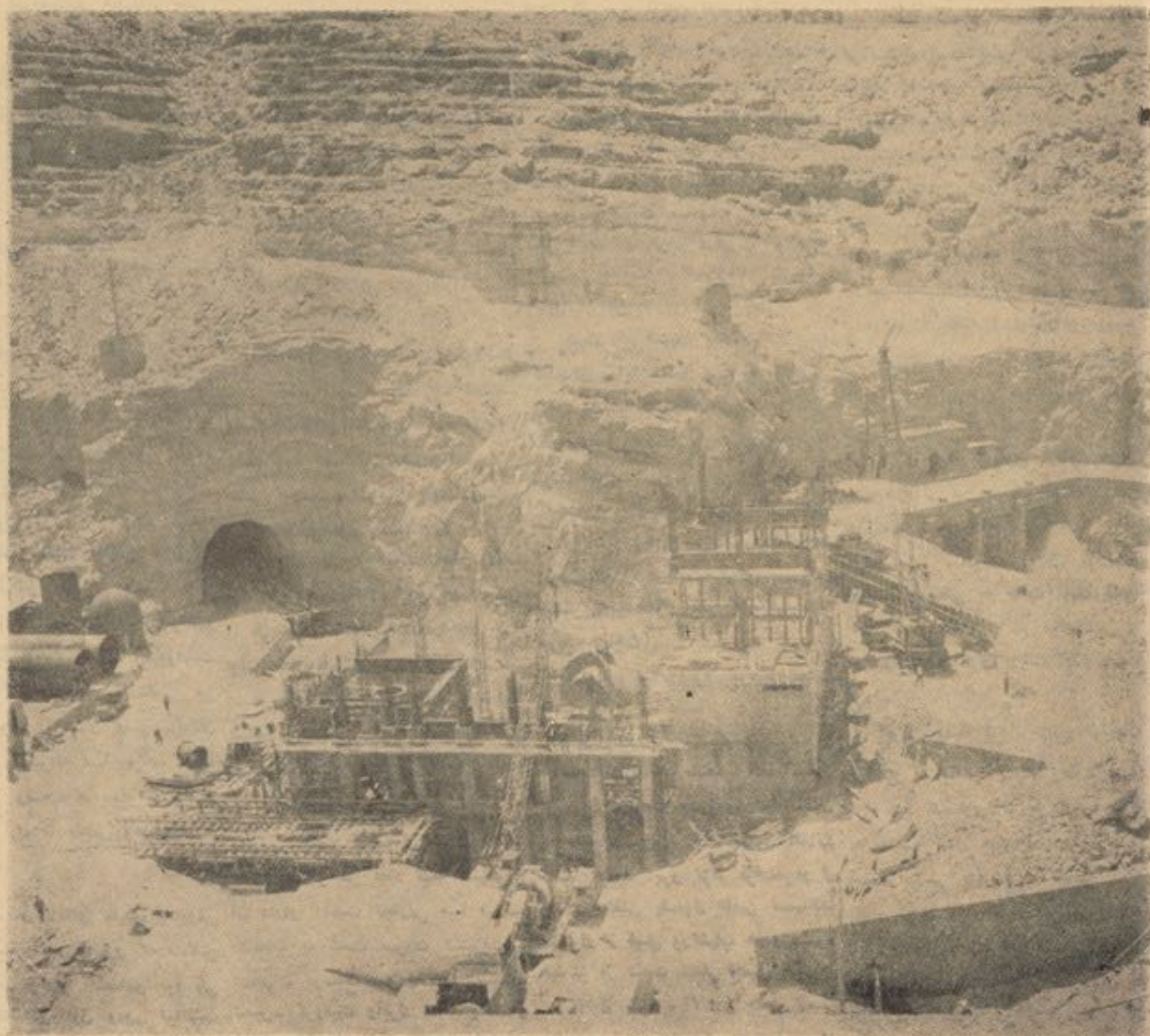
دستگاه تولید برق کجکی در حال امتحان و بسته کاری
