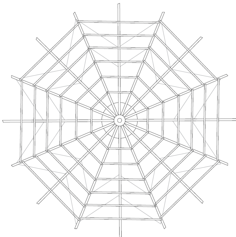
پلان شده بندی پوشش منار غزنی
