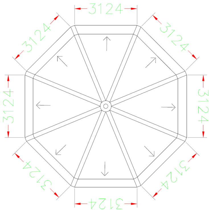
پلان پوشش (آهن پوش) منار غزنی
