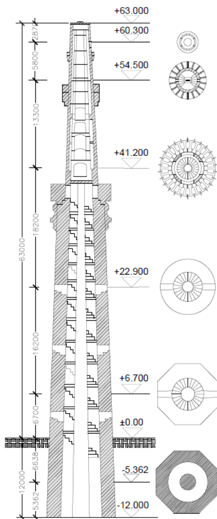
قطع (تراش) ایستاده منار جام در ولایت غور
