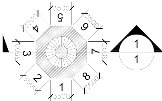
پلان قاعده ای منار جام در ولایت غور
