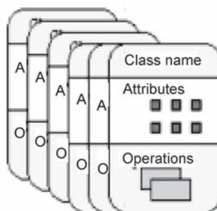
(d) Object-oriented
