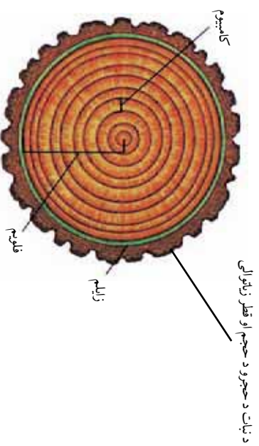
(۶-۸) شکل: مرستېمونه چې د نبات د حجرو د حجم او قطر زیاتوالی سبب کېږي او د ساقې د خوځې مرستېمونه او هغه رېښه چې د نبات د جوړېدو سبب کېږي.
