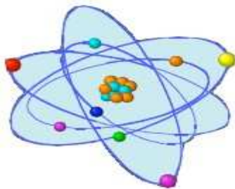
د ډیبرو الکترونو اتوم موډل
