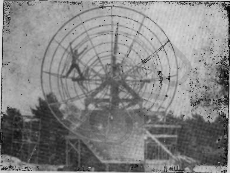
راد یو تلسکوپ
