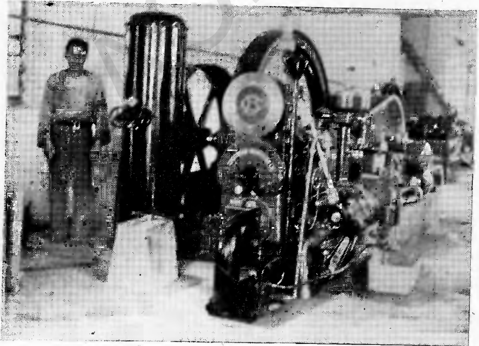
انجن فل پرس فابریکه بشمینہ بافی قندهار
