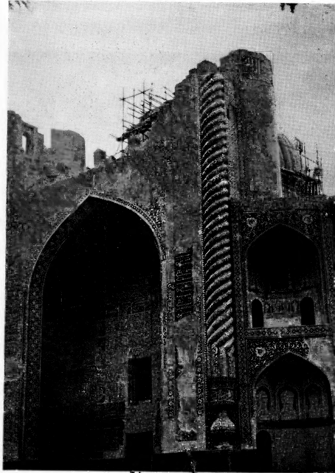
مسجد خواجه ابونصر پارسا در بلخ در مرحله آخر ترمیم
