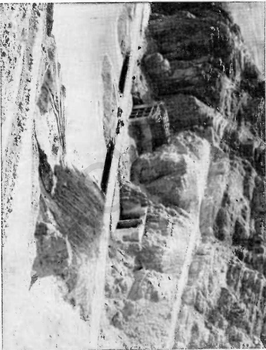
پاك منظره د بنگر بند كچه كې وداخل تونل هاي برق و تونل آبياري در حالت تهدير
