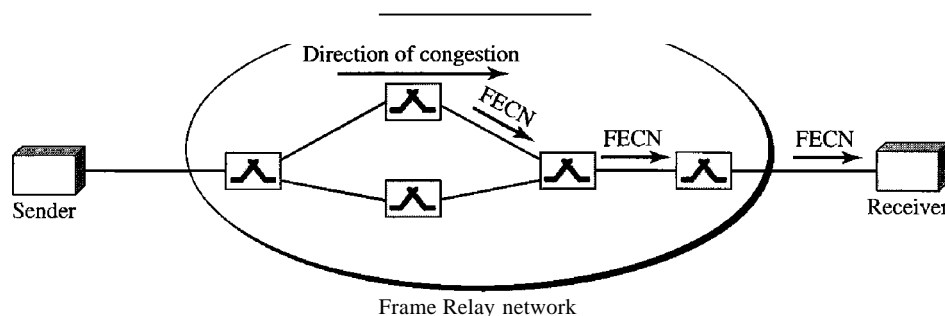
Figure 24.13 FECN
