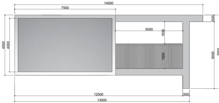
د پوښنښ پاڼې (آخري) مرحلې پلان
