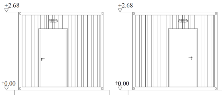
نمای پیشرو و عقب کانتینر حمام تونلی تی آی ام
