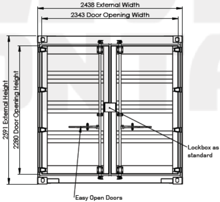
نمای دروازه کانتینر ۱۰ فوت مینی
