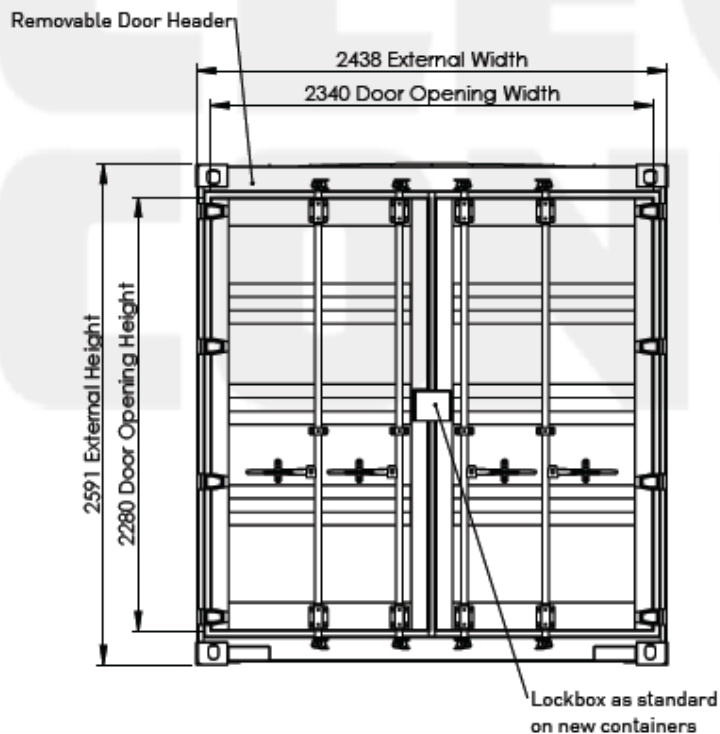
نمای دروازه کانتینر ۲۰ فوت استاندارد سر باز
