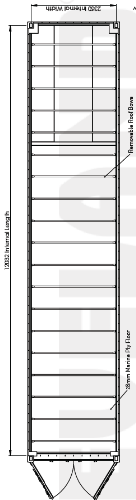
پلان کانتینر ۴۰ فوت ستندرد باز شونده چت
