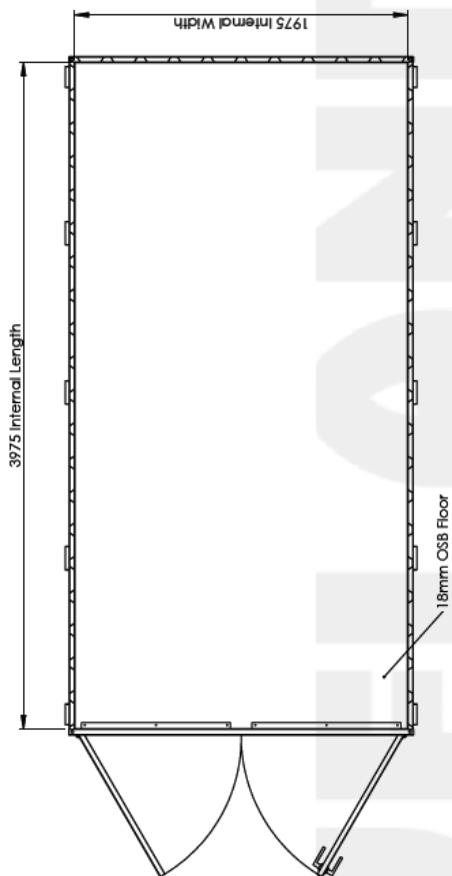
پلان کانتینر فلت پک ۴ در ۲ متر
