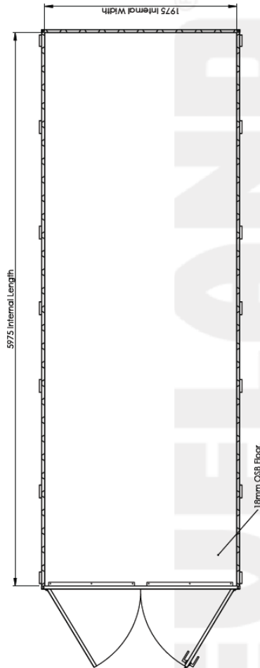
پلان کانتینر فلت پک ۶ در ۲ متر
