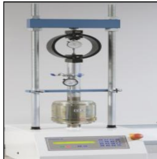
نمونه تست CBR در زیر ماشین فشار
