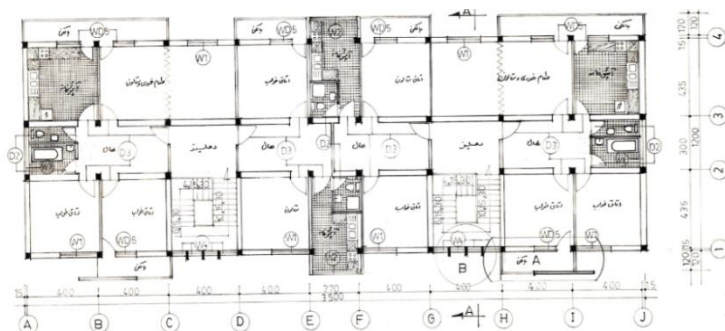
پلان بلاک رهائشی واقع حصه اول خیر خانه ( کابل )
