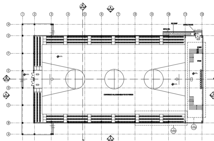
پلان جننازیوم ( ولایت بدخشان )
