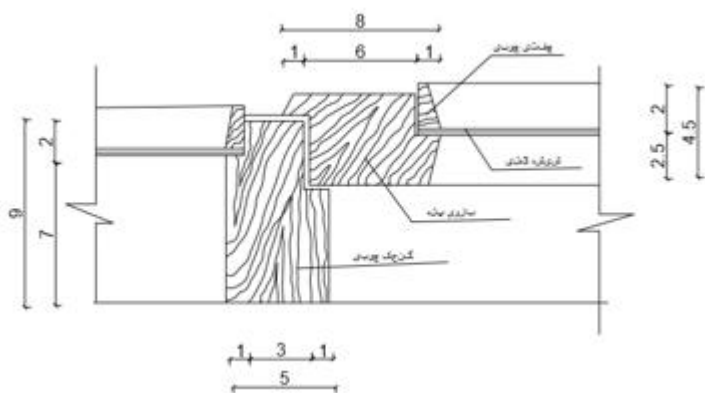
دیتایل D-D
