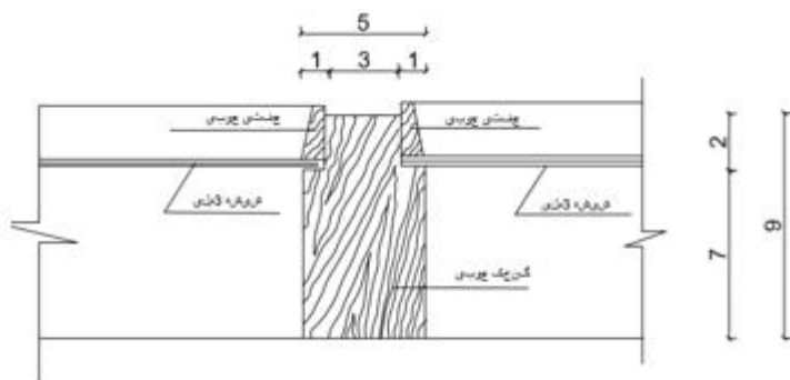
دیتایل E-E
